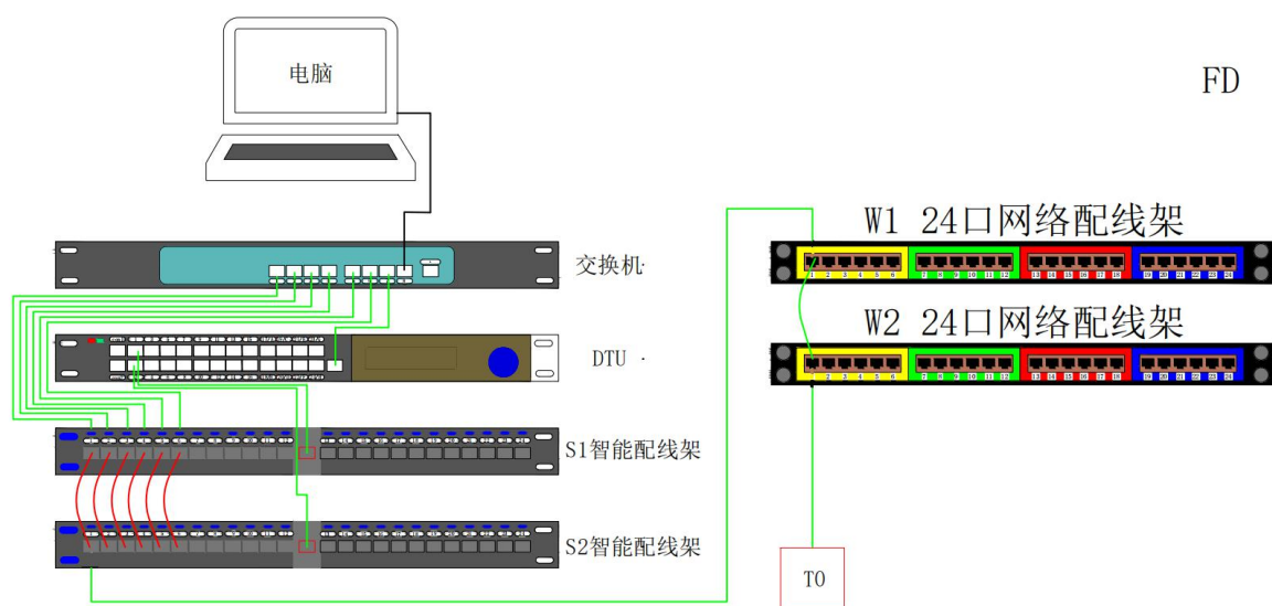
图 14 智能布线管理系统拓扑图
