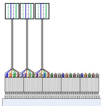
图 13 程控交换机跳线接线示意图
