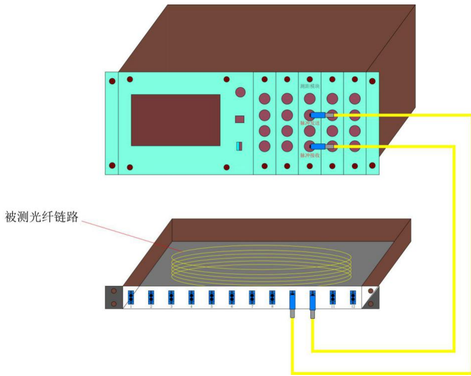
图 10 光纤链路长度测试原理图
